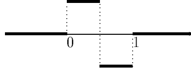
Рис.2. Всплеск Хаара.
