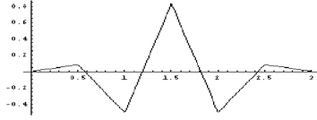
Рис.1. График \psi^2(t) .
