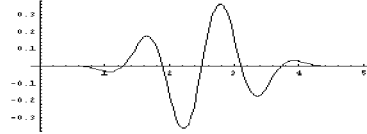
Рис.2. График \psi^3(t) .
