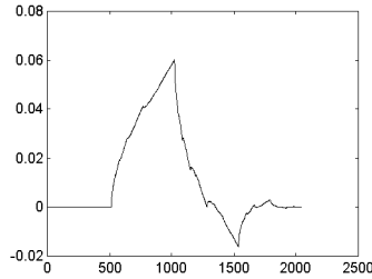
Рис.1. График \varphi^{D,2}(t) .
