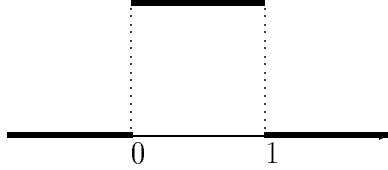
Рис.1. Масштабирующая функция Хаара.
