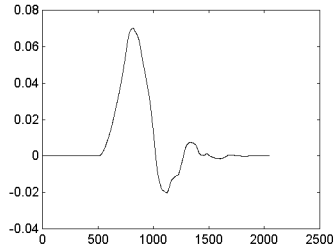
Рис.1. График \varphi^{D,4}(t) .
