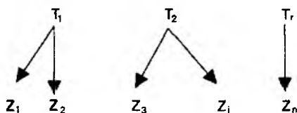
Рис. 7.2. Схема соотношений между теоретическими понятиями ( T ) и эмпирическими индикаторами ( z )
