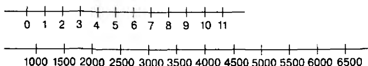
Рис. 5.5. Примеры интервалов на числовой оси, отвечающих «ячейкам», используемым при построении установочной шкалы Терстоуна
