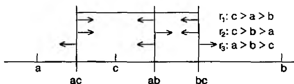
Рис. 9.4. Поиск геометрических мест идеальных точек трех гипотетических респондентов
