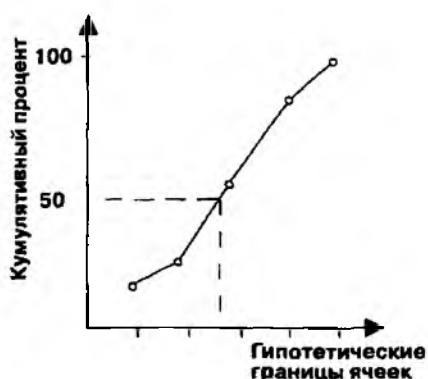
Рис. 5.7. Расчет медианы при условии откладывания кумулятивного процента от правого конца интервала
