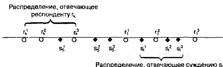
Рис. 5.3. Распределения, отвечающие отдельным респондентам (○) и суждениям (◆)
