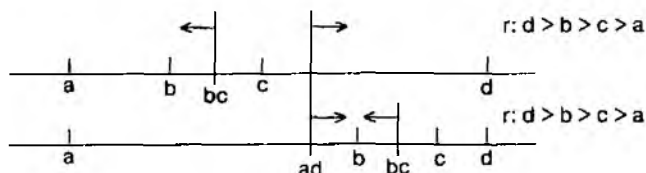
Рис. 9.6. Иллюстрация зависимости возможности построения шкалы от соотношения длин интервалов между точками, отвечающими шкалируемым объектам
