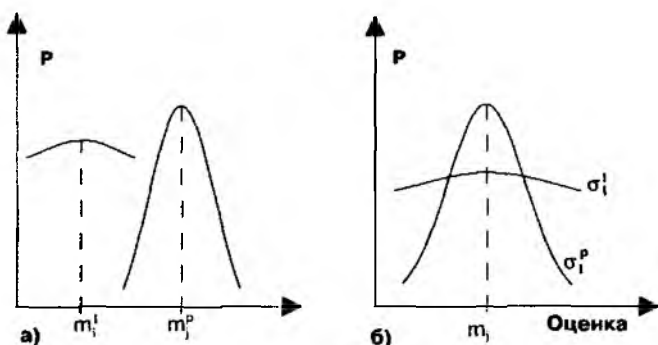
Рис. 6.4. Распределения оценок i -го объекта, данных l -м и p -м респондентами: а) — с разными средними и разными дисперсиями; б) — с одинаковыми средними, но разными дисперсиями
