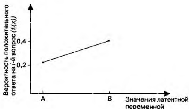
Рис. П2.1. График i -го вопроса f_i(x)
