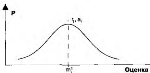
Рис. 6.2. Нормальное распределение оценок i -м респондентом j -го объекта
