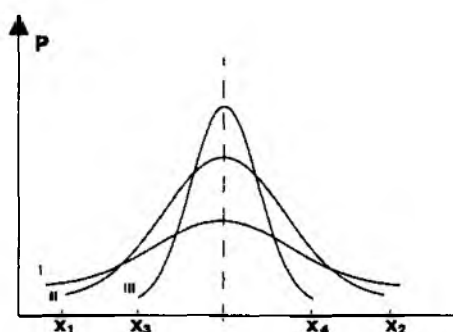
Рис. 6.3. Нормальные распределения оценок i -м респондентом i -го объекта при разных дисперсиях
