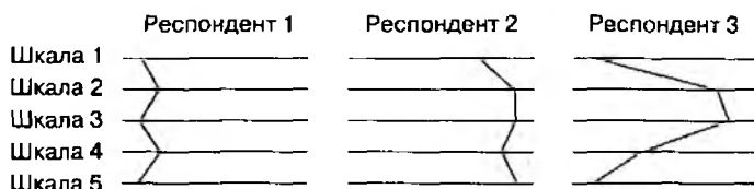
Рис. 8.1. Примеры профилей, полученных с помощью техники СД
