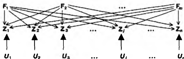
Рис. 7.1. Схема соотношений между наблюдаемыми признаками ( z_1, \dots, z_n ) и латентными факторами: общими ( F_1, \dots, F_m ) и специфическими ( U_1, U_2, \dots, U_n )
