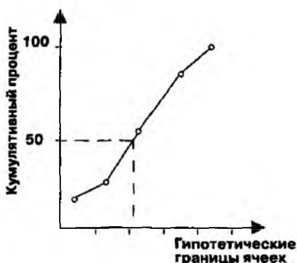
Рис. 5.6. Расчет медианы при условии откладывания кумулятивного процента от середины интервала
