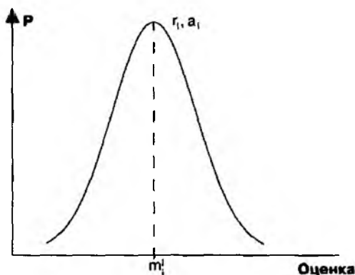
Рис. 6.1. Нормальное распределение оценок l -м респондентом i -го объекта
