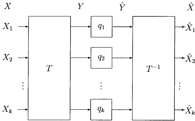
Fig. 4. Transform code.
