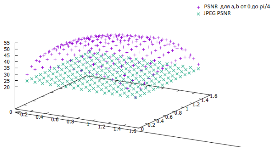
Рис.2. Результат тестирования для портретного снимка.
