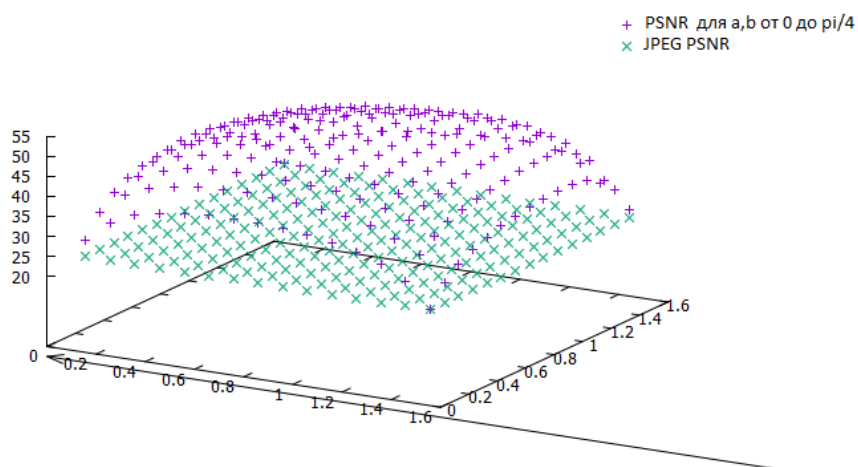
Рис.3. Результат тестирования для пейзажного снимка.
